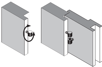
Otočitel'né závěsy dveří Otočitel'né závěsy dverí
